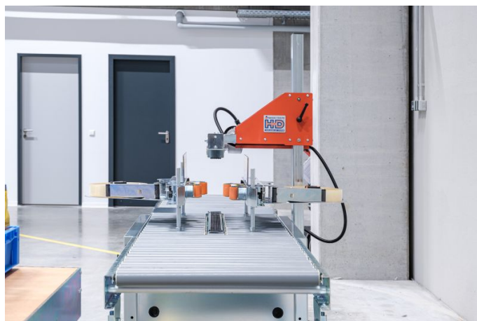
Blick einlaufseitig auf den Kartonverschleißer ST-10.
