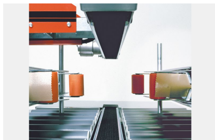
Die oben und unten liegenden Antriebskassetten garantieren einen zuverlässigen Transport.
