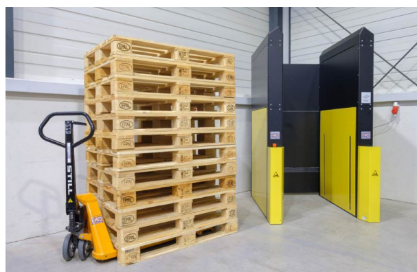
Komplett-Entnahme oder -Zuführung eines ganzen Stapels ist ebenfalls möglich
