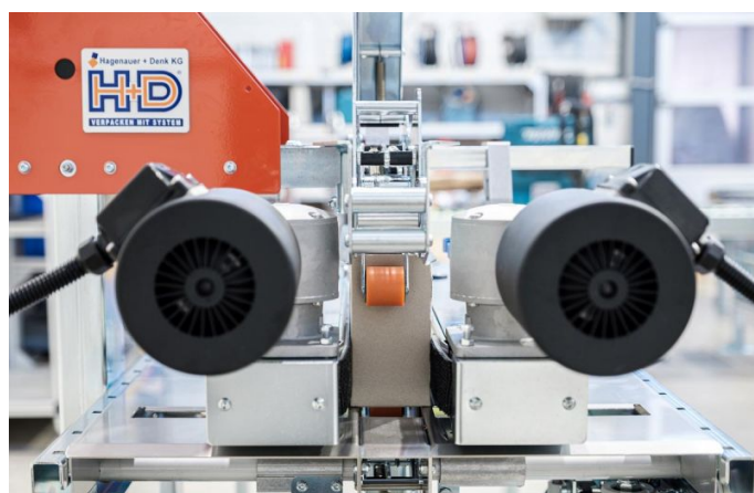
Sicherer Verschluss schon ab 60 mm Kartonbreite.
