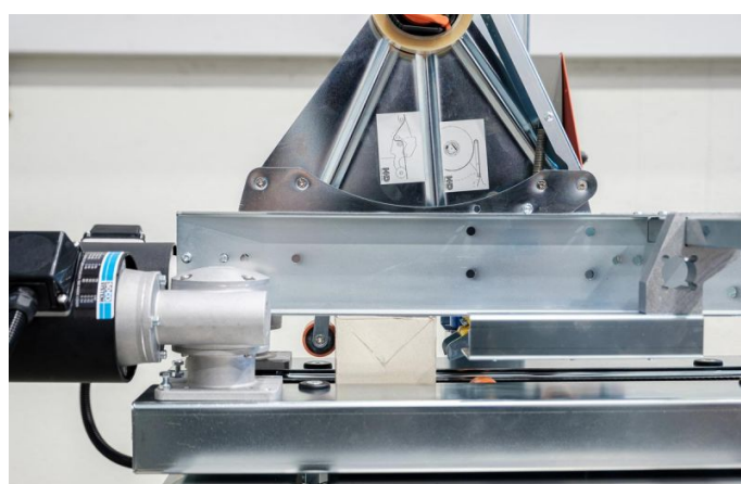
Andruckrollen garantieren einen sicheren und faltenfreien Klebebandauftrag.
