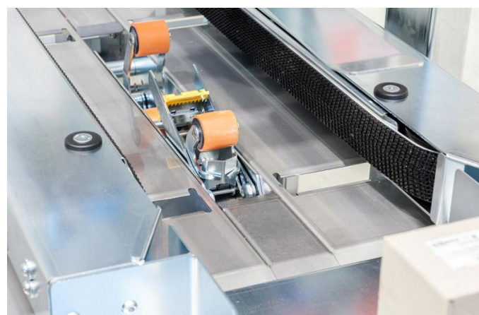
Plattenbettung für sicheren und ruhigen Transport von Kleinstkartons.
