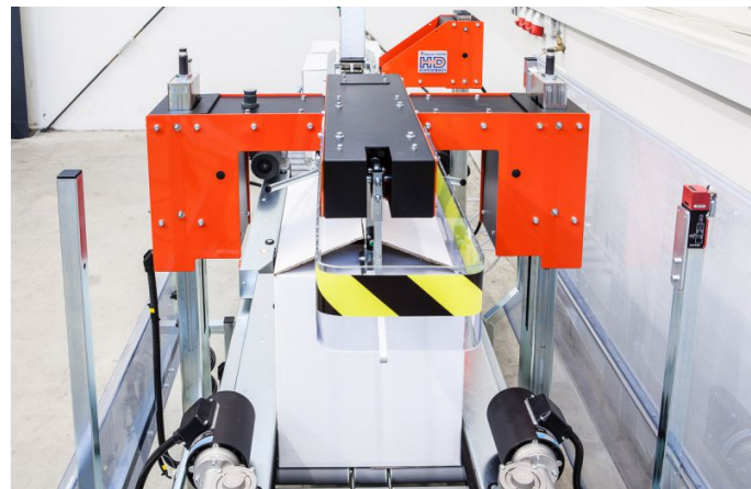
Einfaltmechanismus mit Schutzbügel
