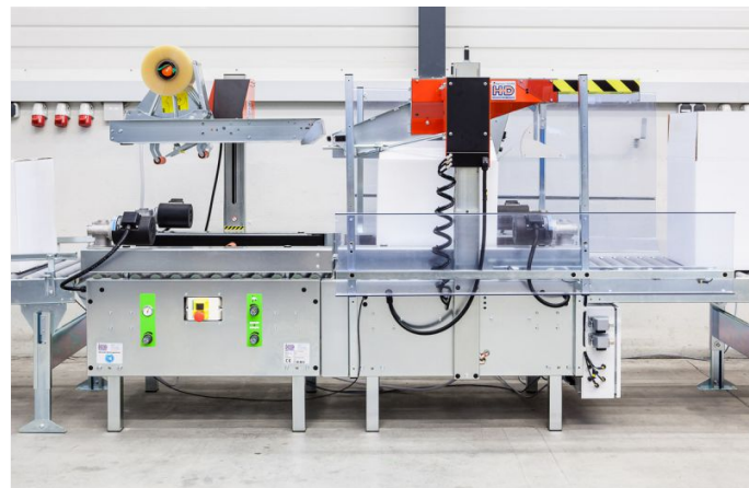
Automatische Übergabe eines Kartons von dem Deckelklappenfalter zum Kartonverschleißer
